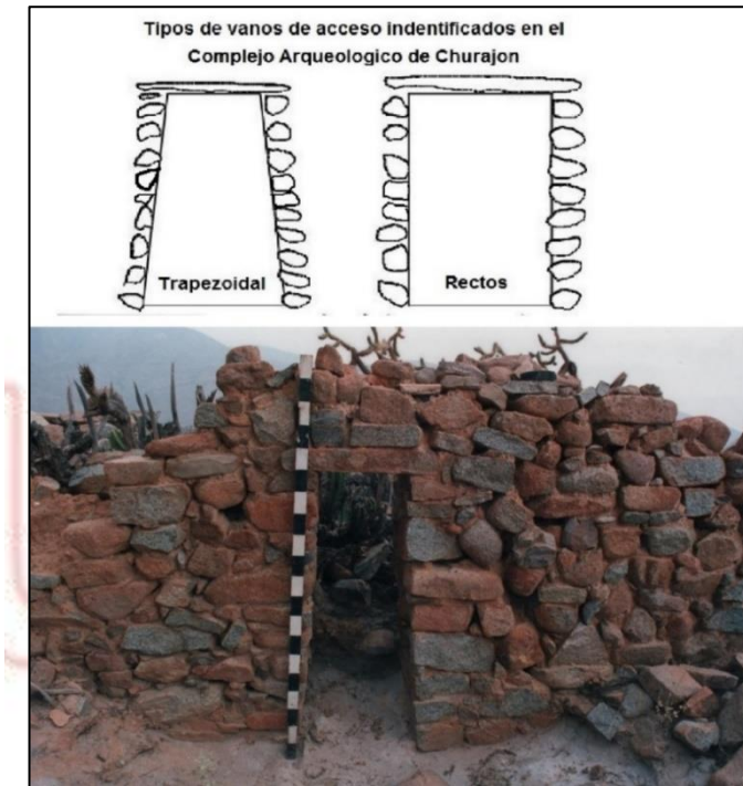
Fig. 15: Arquitectura Churajón
